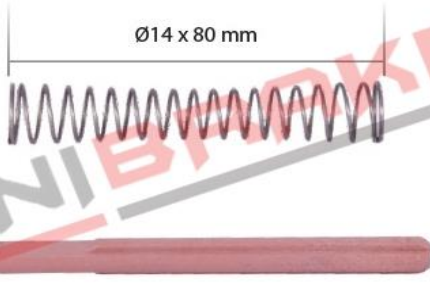
7243 / Caliper Visual Indicator ELSA 2 Type
