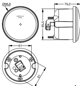
Bus Tail Fog Lamp (12 LEDs) Otobüs Arka Sis Lambası (12 Ledli)
