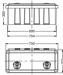
Trailer Tool Box 42 Liters Dorse Alet Çantası 42 Litre
