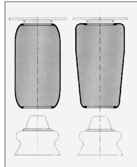
zylindrischer Rollbalg
