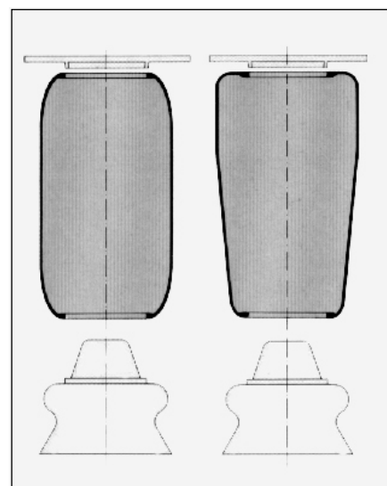
Enveloppe Cylindrique
