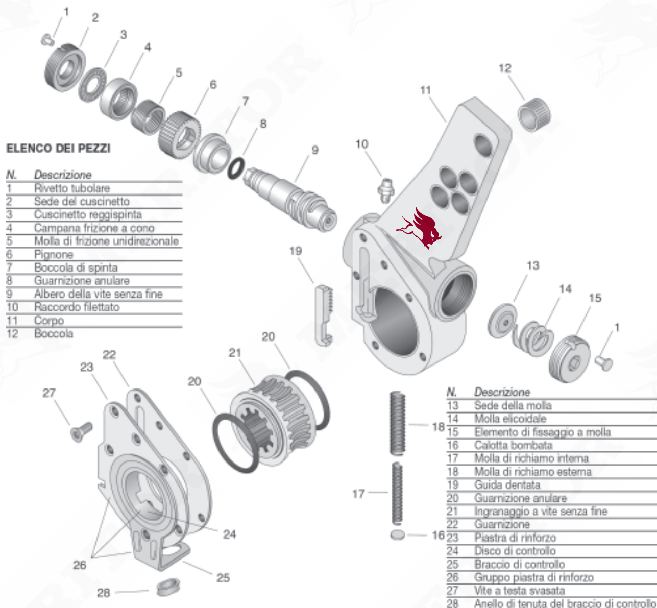
STAFFA DEL TIPO A SELLA
