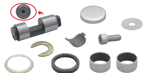
MTX-4238 Camshaft Kit Zestaw naprawy
