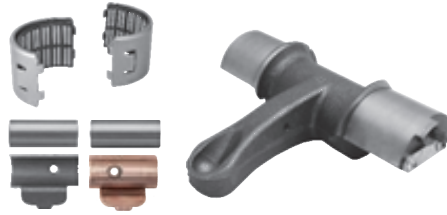
MTX-7042 Repair Kit Zestaw naprawczy CMSK.5.14 | 3092258 | 21109753
