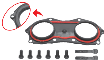
MTX-5271 Mech. Cover (SN6/SK7) Płyta dolna zacisku
