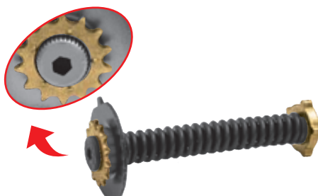
MTX-5027S Pinion Shaft Walek pomocniczy reg. CKSK.10.4
