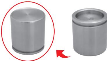
MTX-4017 Piston - F/B (68x73,5 mm) Tłok ham. (68x73,5 mm)
