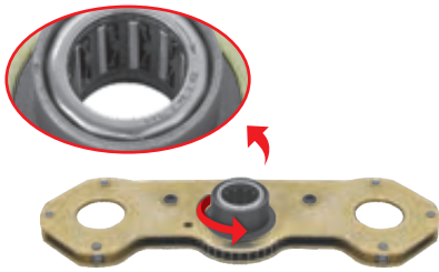
MTX-7124 Adjusting Mechanism Mechanizm samoregulacji
