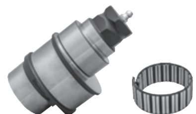
MTX-7914 Camshaft Set Wałek mimośrodowy z łożyskiem
