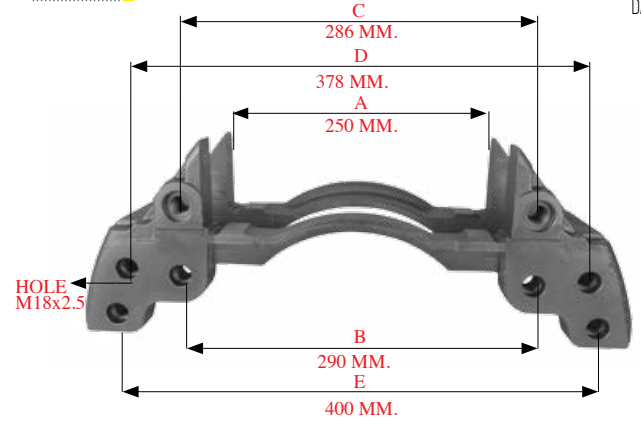
190109 > BALATA TAŞIYICI / CARRIER
