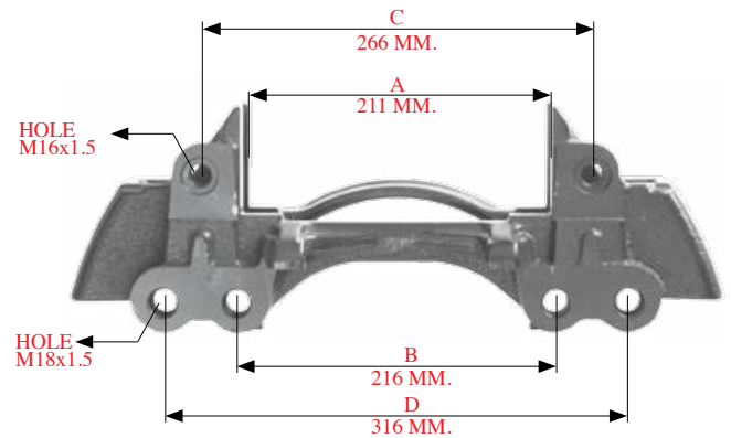
190112 > BALATA TAŞIYICI / CARRIER
