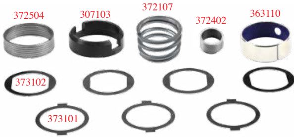
340403 AYAR DIŞLİSİ KİLİT TAKIMI - R - CLUTCH SYSTEM - R -
