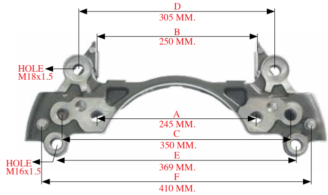
390103 > BALATA TAŞIYICI / CARRIER
