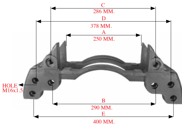
190111 > BALATA TAŞIYICI / CARRIER
