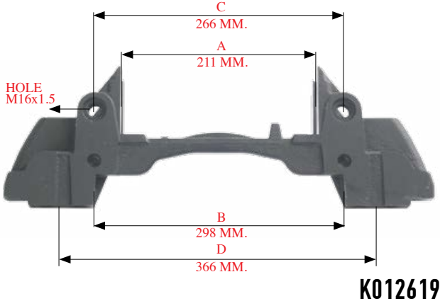
190101 > BALATA TAŞIYICI / CARRIER SK7...
