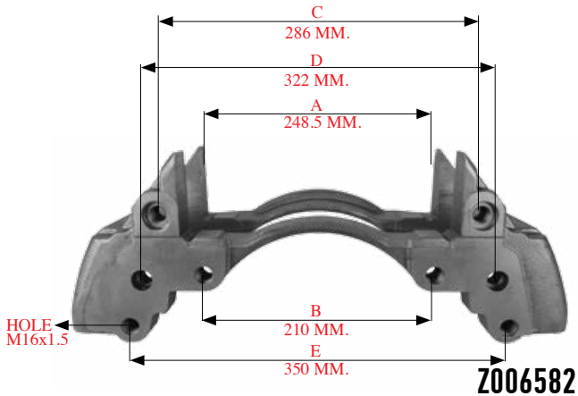
190105 > BALATA TAŞIYICI / CARRIER
