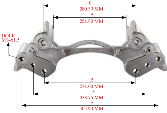
390101 > D3 BALATA TAŞIYICI D3 CARRIER
