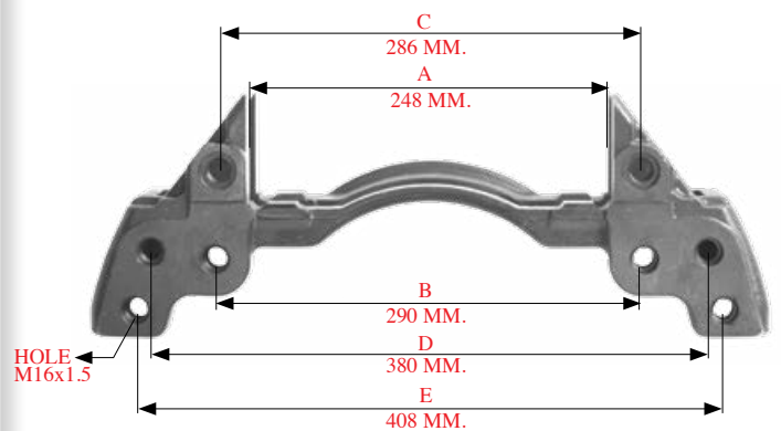
190115 > BALATA TAŞIYICI / CARRIER
