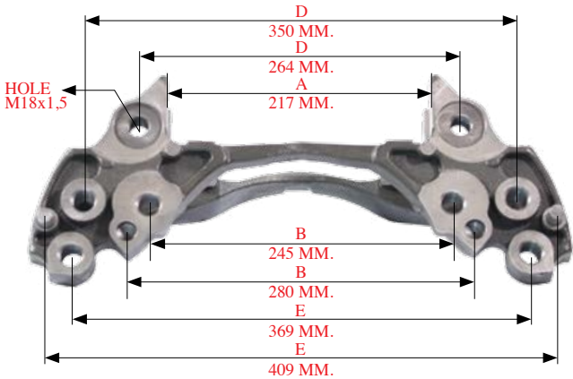
390105 > BALATA TAŞIYICI / CARRIER
