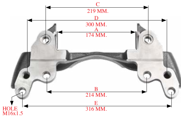
190113 > BALATA TAŞIYICI / CARRIER
