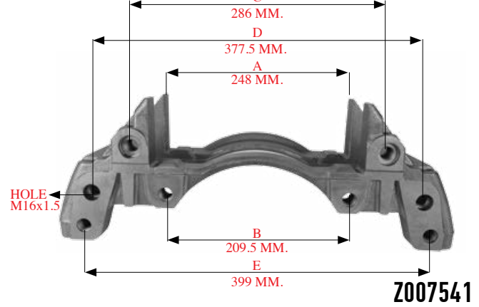
190102 > BALATA TAŞIYICI / CARRIER
