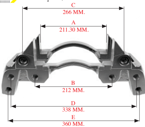
190107 > BALATA TAŞIYICI / CARRIER
