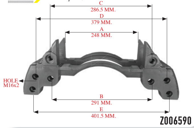
190103 > BALATA TAŞIYICI / CARRIER
