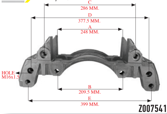
190102 > BALATA TAŞIYICI / CARRIER
