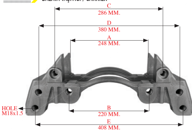
190104 > BALATA TAŞIYICI / CARRIER
