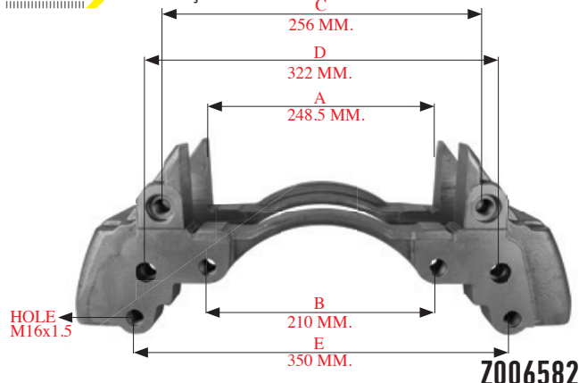
190105 > BALATA TAŞIYICI / CARRIER
