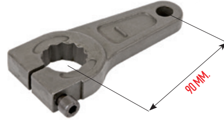
314103 > KALİPER ŞAFT LEVYESİ CALIPER SHAFT LEVER
