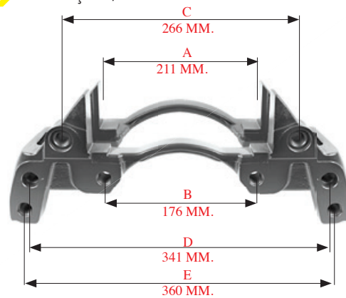
190108 > BALATA TAŞIYICI / CARRIER
