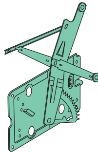
OFM/174 d-rh-rechts OFM/175 s-lh-links elettrico, senza motorino electric, without motor elektrisch, ohne Motor
