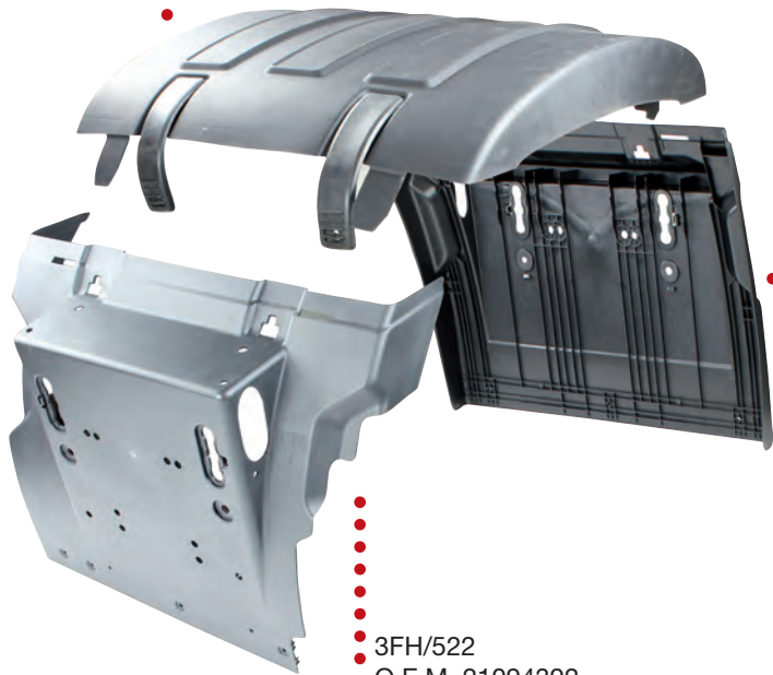
vista esterna - external view Außenansicht
