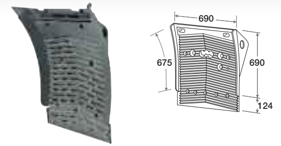
H. 124 TGX/540 O.E.M. 81664106609
