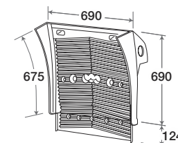
H. 217 TGX/518 O.E.M. 81664106604
