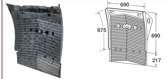
H. 217 TGX/512 O.E.M. 81664106601
