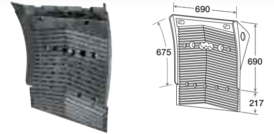
H. 217 TGX/512 O.E.M. 81664106601
