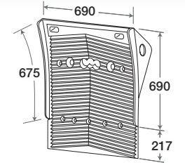
H. 217 TGX/512 O.E.M. 81664106601
