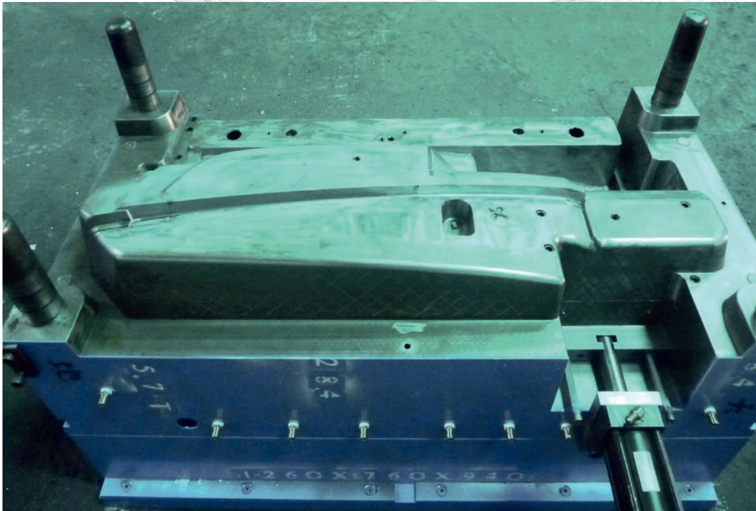
▲ IT Stampo in acciaio a iniezione per la produzione di deviatore aria Daf LF euro 6 EN Steel injection moulding for the manufacturing of the air deflector for the DAF LF Euro6 DE Spritzgusswerkzeug aus Stahl für die Herstellung des Luftabweisers des DAF LF Euro6
