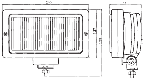
SL 2221 KROM NİKEL - CHROME SİS LAMBA - FOG LAMP
